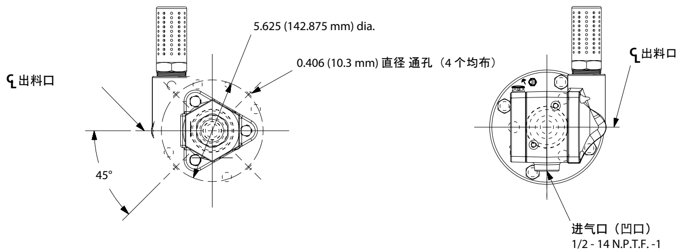
底视图
