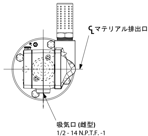
上部図
