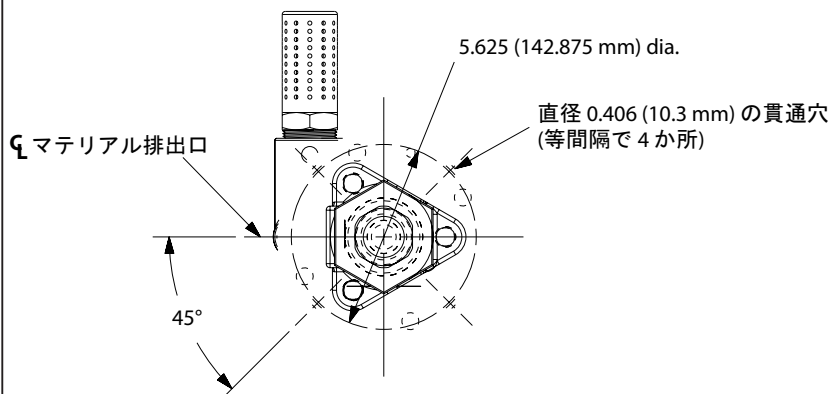
下部図
